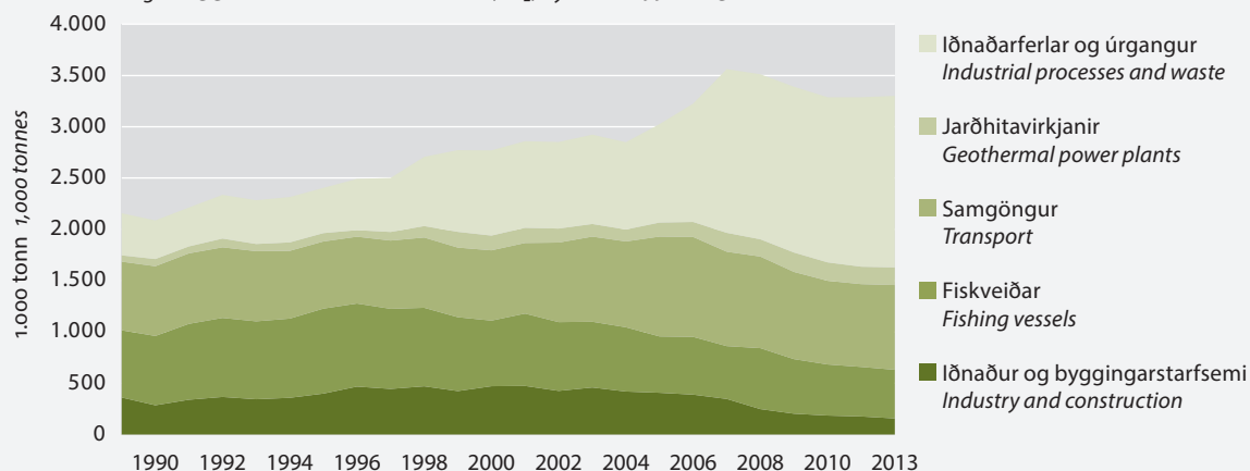
Mynd 23.3 Útstreymi koldíoxíðs (CO 2 ) eftir uppruna 1990–2013
